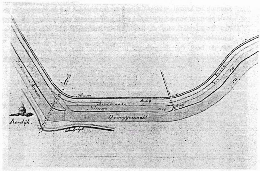
Figuur 1. Fragment van de ontwerptekening voor de aanleg van het Noordhollandsch Kanaal. Rijksarchief Haarlem, Kaartenarchief Rijkswaterstaat, voor 1850.
